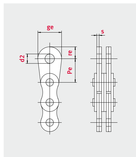
Koło powrotne: bmin = całkowita szerokość łańcucha (B x 1.05) Idler wheel: bmin = overall width of chain (B x 1.05)
