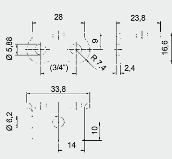
Für Kette M 128 A SL: Form 202.8
