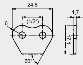
Für Kette L 85 SL: Form 106.0 Führungslasche für Innenglieder
