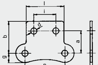
101.2 für Langgliederketten
