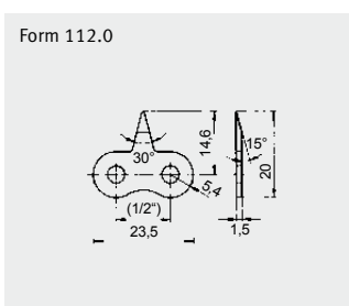
Form 112.0 FL85SL mit 112.0: Art. 50002138
