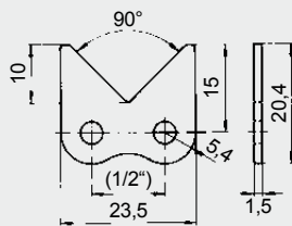
Für Kette L 85 SL: Form 110.0
