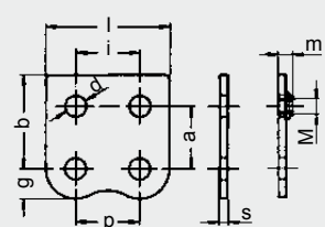
103.32 mit Gewindeeinsatz
