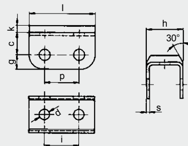
Form 303.9 mit Gummiauflage
