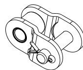
Normbezeichnung L Gekröpftes Glied mit Splintverschluss
