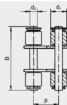
Steckglied
