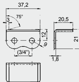
Für Kette M 127 SL: Form 203.8
