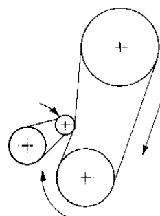
RICHTIGE MONTAGE
