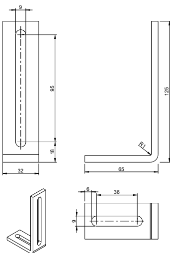
Befestigungswinkel 01
