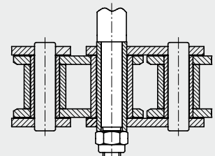
iwis POChain-S
