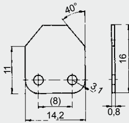
Für Kette G 52: Form 103.7
