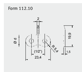
Form 112.10 Mehrere Varianten
