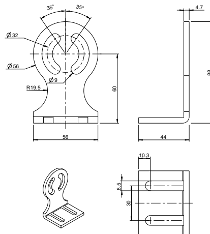
Befestigungswinkel 02
