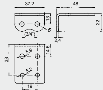
Für Ketten M 128 A SL/M 128 A SB, Form 222.2
