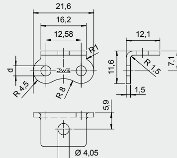
Für Kette P83V: Form 220.15
