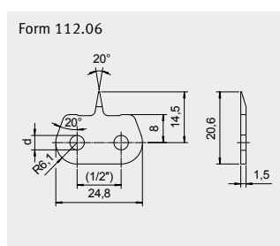
Form 112.06 FD85SL mit 112.06: Art. 50019757
