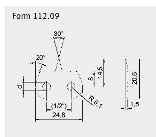
Form 112.09 FD85SL mit 112.09: Art. 50028230
