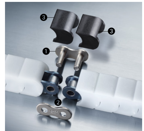
Verbindungsglied: gleiche Abmessungen wie Kette
