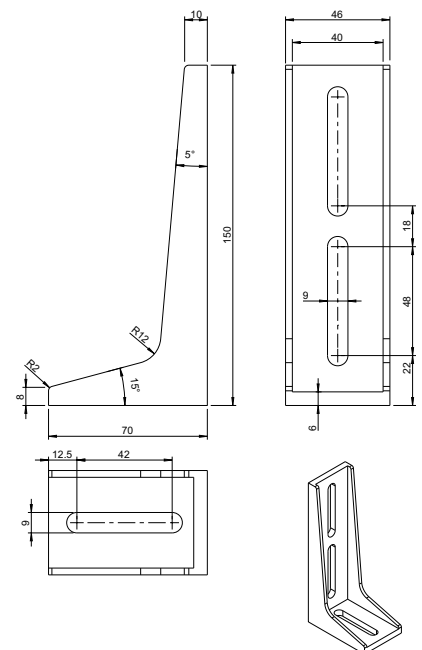
Befestigungswinkel 03
