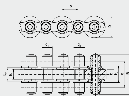
Bauform M mit seitlichen Scheiben
